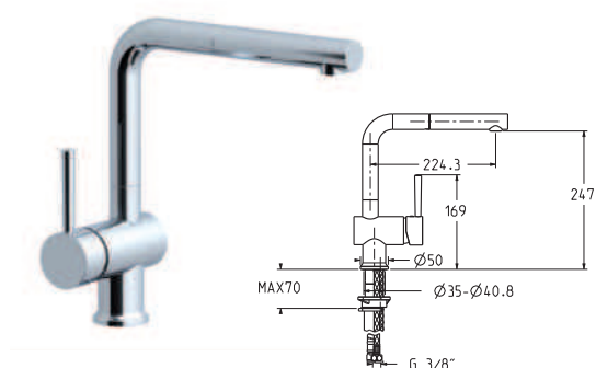
art. 0410 DOCCIA ESTRAIBILE
